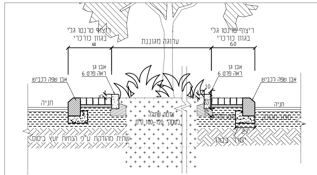
חתך A-A
