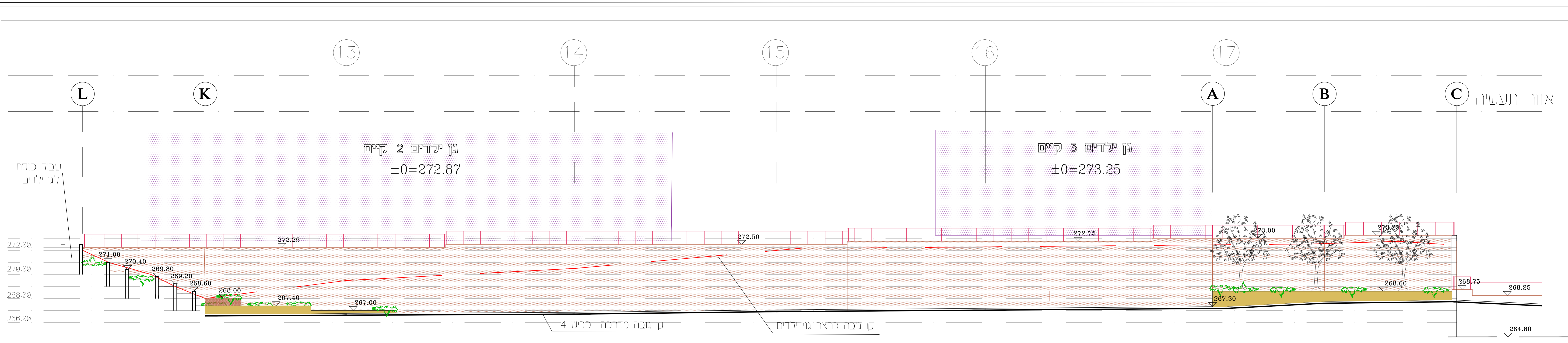
פריסת קיר L-K-A-B-C תומך אזור גני ילדי לאורך כביש 4
