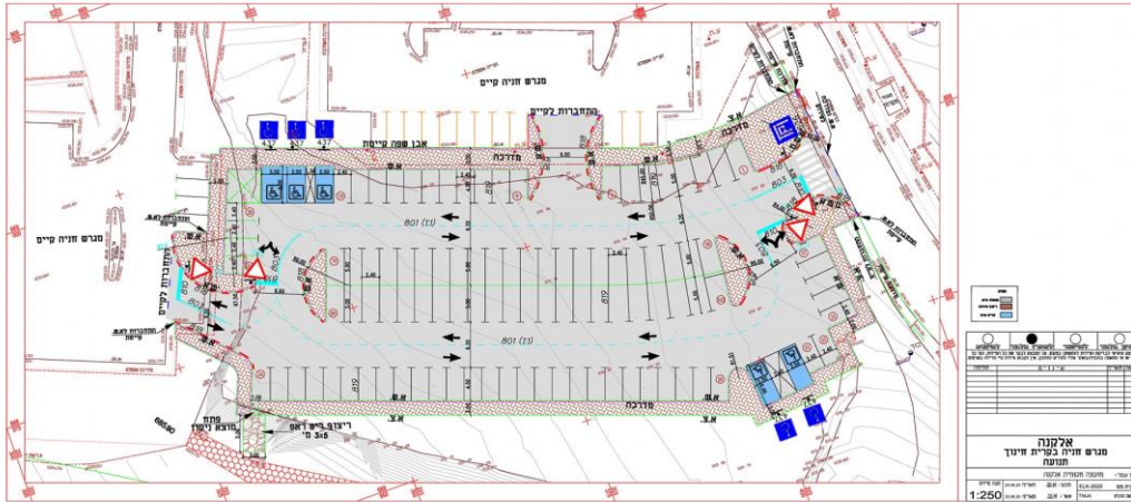
תוכנית החניה החדשה
